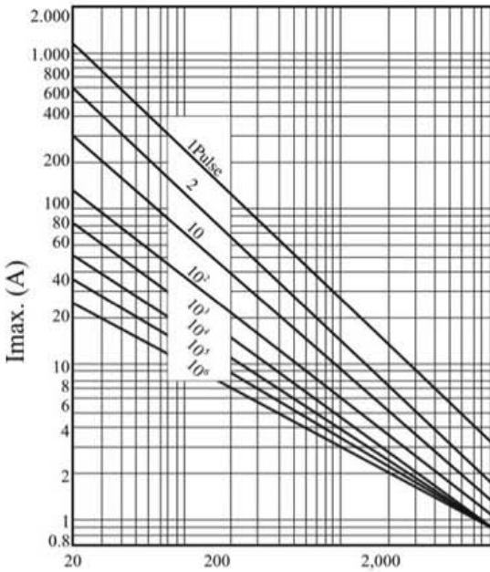
JVR07N820K~JVR07N821K
